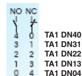
Kontaktblock-Frontmonterat
